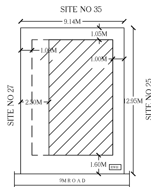
SITE PLAN 1:200
