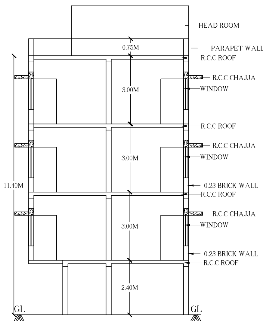
SECTION A-A
